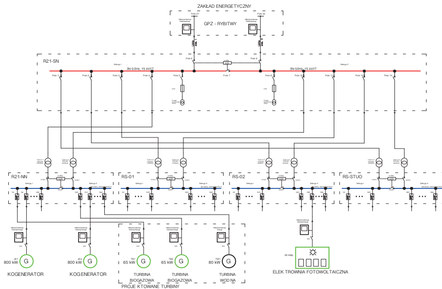
Schemat układu elektrycznego oczyszczalni Płaszów po realizowaniu projektu
