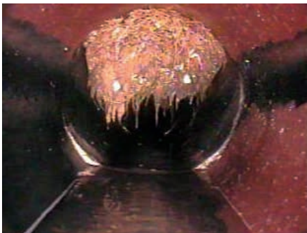
Ryc. 6. Osad stały w nowym przewodzie kanalizacyjnym [3]
