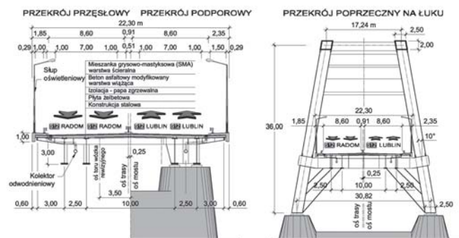
Ryc. 5. Przekroje poprzeczne prześel na terenie zalewowym i przęśla nurtowego
